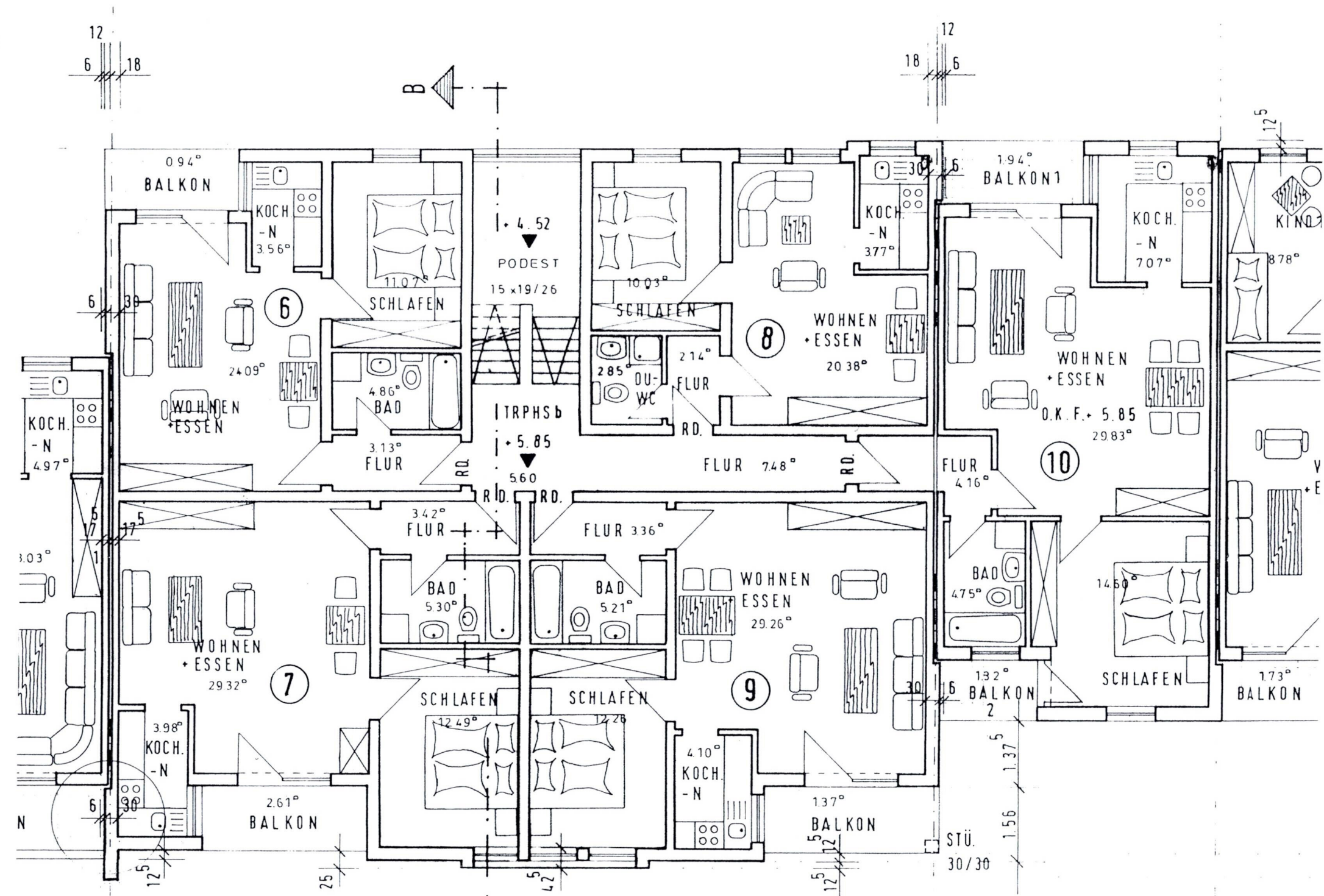
Grundrissplan 2. Obergeschoss: (nicht maßstabsgerecht)
