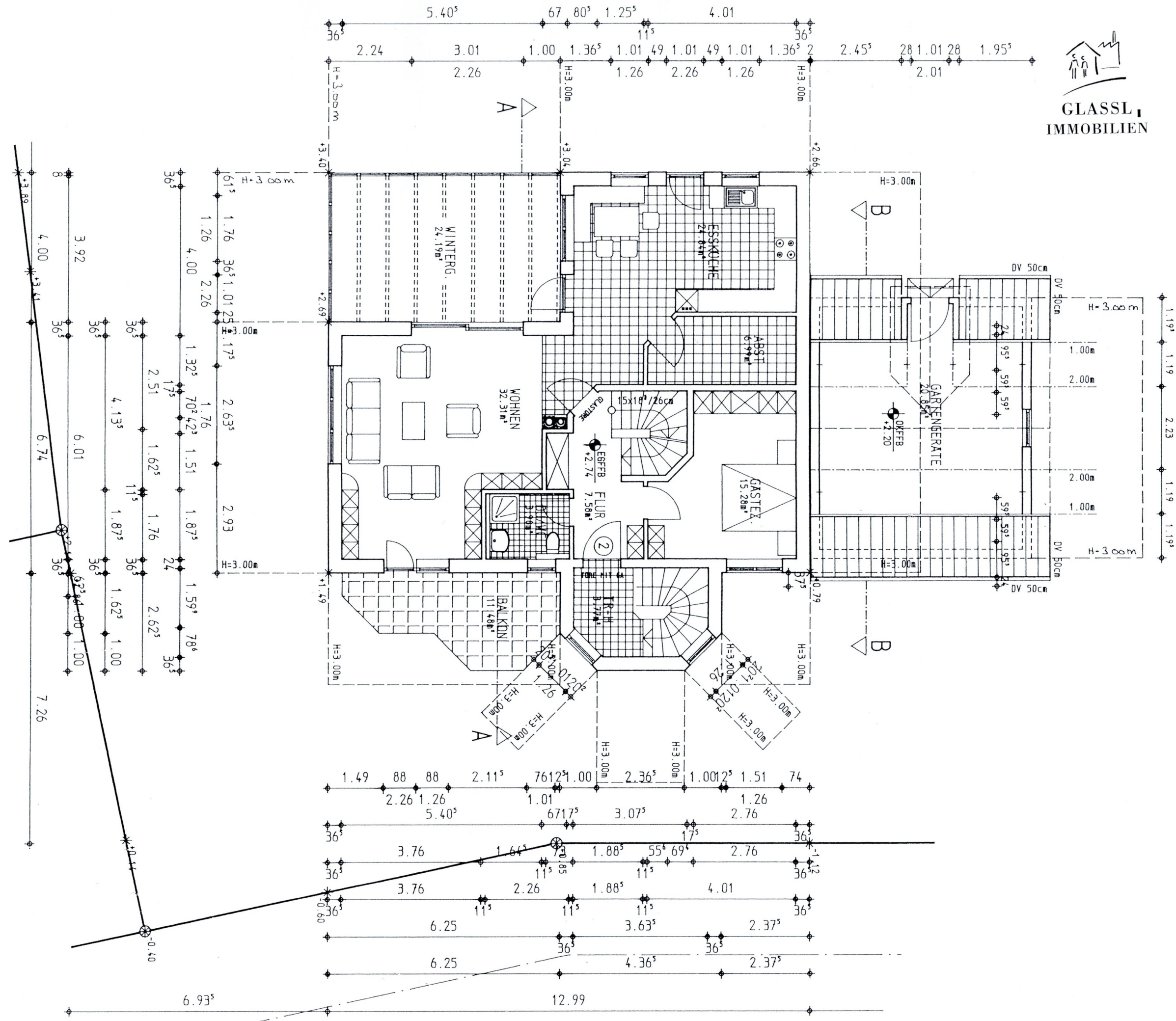
Grundrissplan: Erdgeschoss (nicht maßstabsgerecht)
